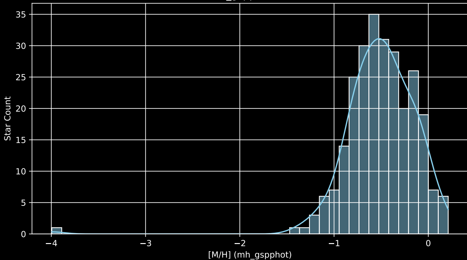
GALAH DR4 Field: [1223] [M/H] (mh_gspphot) (n= 261)
