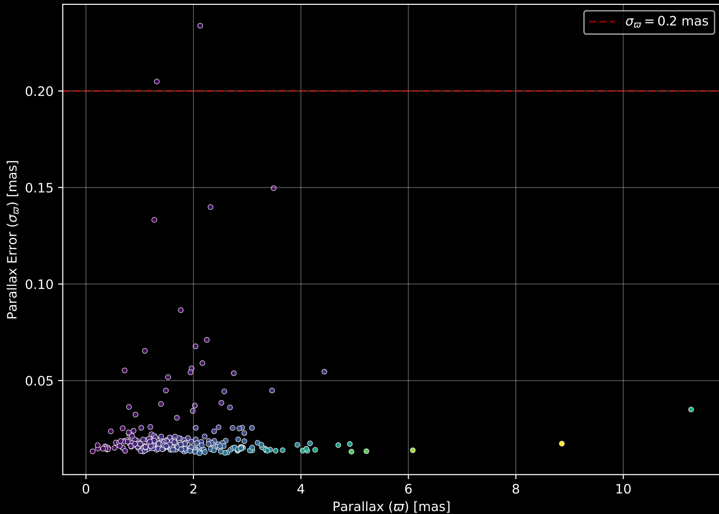
GALAH DR4 Field: [1223] Parallax Quality (n= 261)
