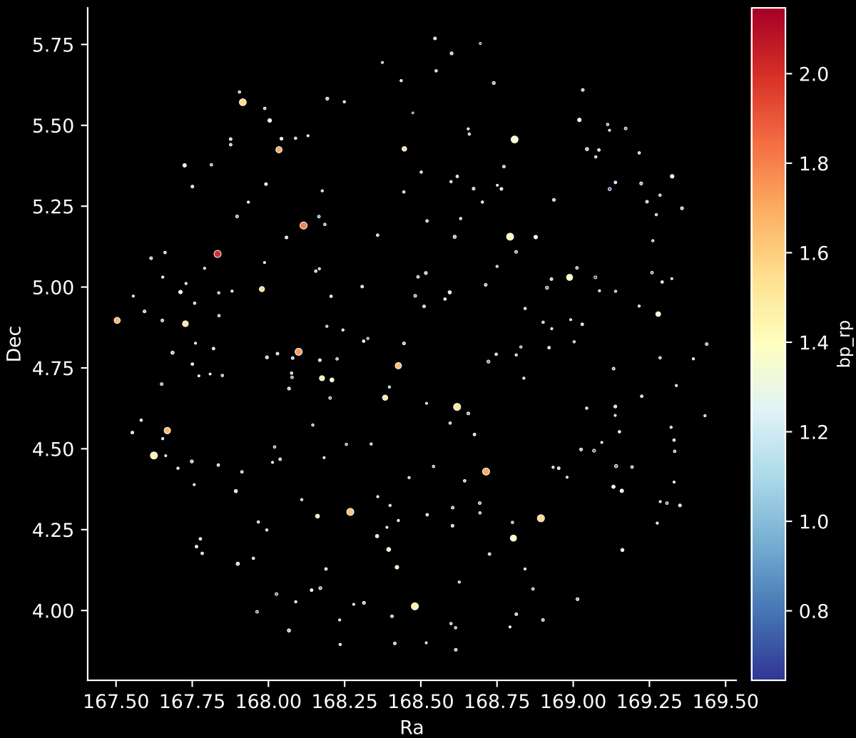
GALAH DR4 Field: [1223] Stars: 261
