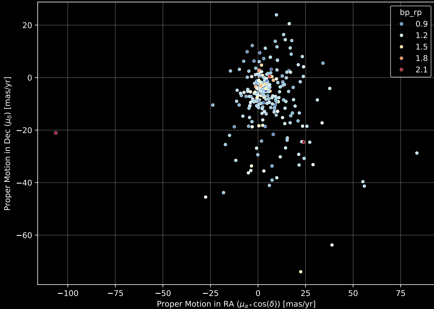
GALAH DR4 Field: [1223] Proper Motion Diagram (n= 261)
