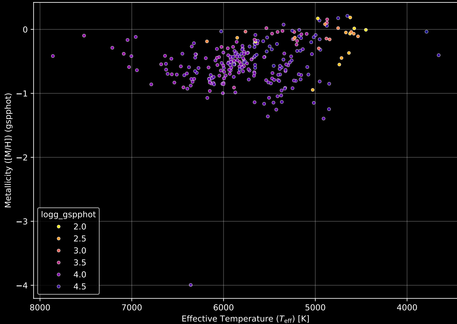
GALAH DR4 Field: [1223] Stellar Population Parameters (n= 261)
